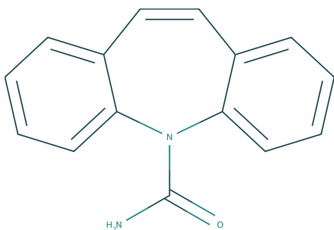
ساختار مولکولی کاربامازپین
